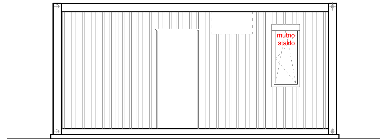
PROČELJE SJEVEROZAPAD
