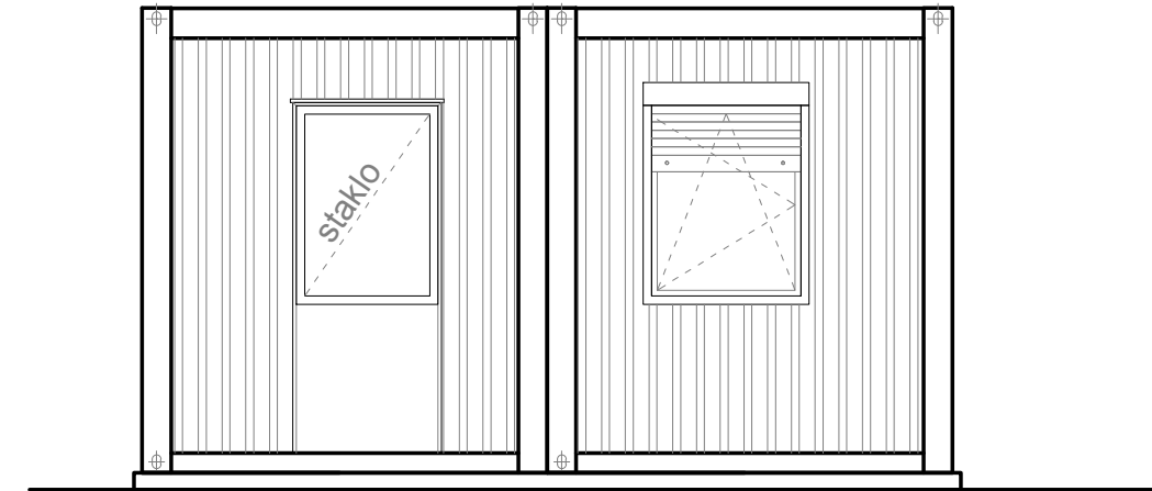
PROČELJE SJEVEROISTOK
