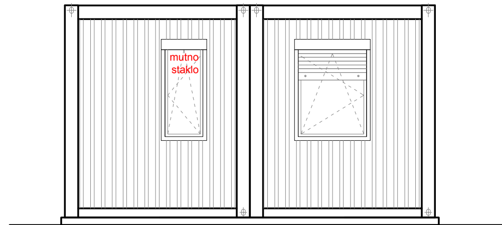
PROČELJE JUGOZAPAD
