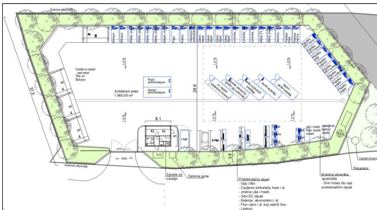
Slika 4: Izgled reciklažnog dvorišta – varijantno rješenje (izvor: „Hidroplan“ d.o.o. za izgradnju i konzalting Zagreb)
